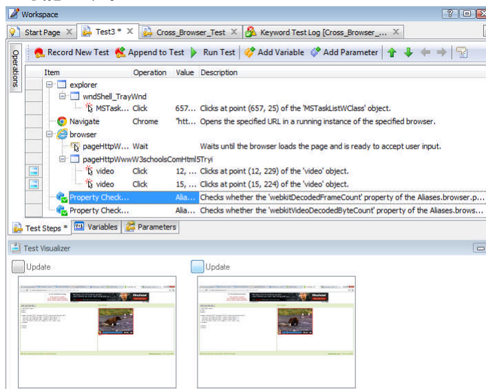
HTML5 オブジェクトのテスト
